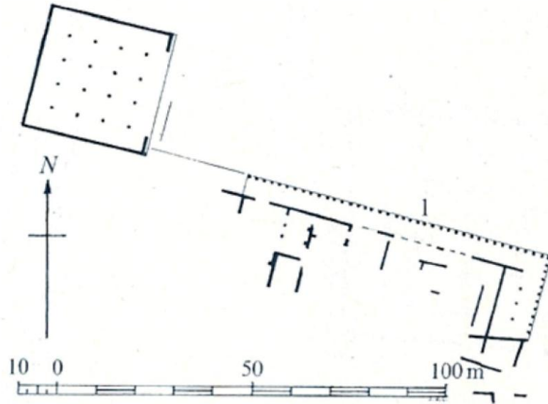
Şekil 22: Argos Agorası Güney Stoası (J. J Coulton 1976, Fig.50)
