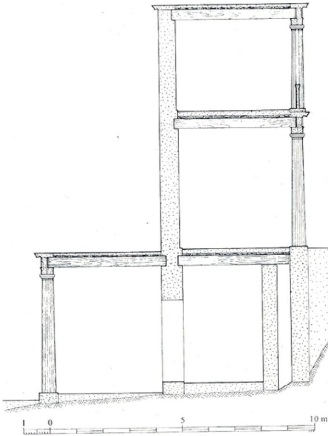
Şekil 30: Bergama, Aşağı Agora güney kanat (J. J Coulton 1976, Fig.14)
