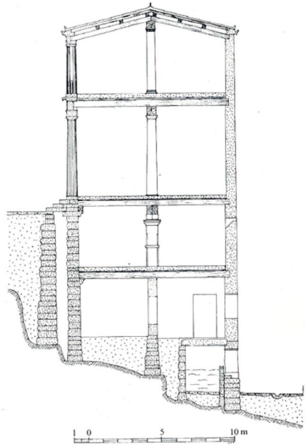
Şekil 31: Assos Güney Stoası (J. J Coulton 1976, Fig.15)
