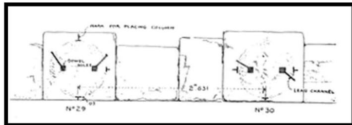
Şekil 43: Stylobat üzerindeki tutturma delikleri ve akıtma kanalları (Clarke, Bacon, Koldewey 1902: 33,5)
