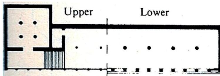
Şekil 21: Atina Asklepios Batı Stoası (J. J Coulton 1976, Fig.25)
