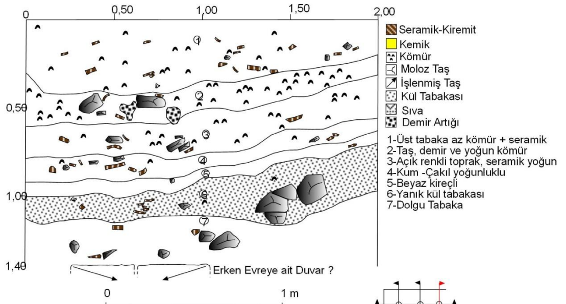
Ölçek: 1/10 Şekil 60: Kuzey Stoa, Alan 1 Profil 7 - Doğu Profili
