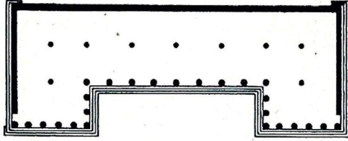
Şekil 18: Atina, Zeus Stoası (J. J Coulton 1976, Fig.23)
