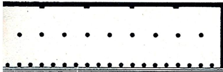
Şekil 17: Argos Kutsal Alanı Güney Stoası (J. J Coulton 1976, Fig.21)
