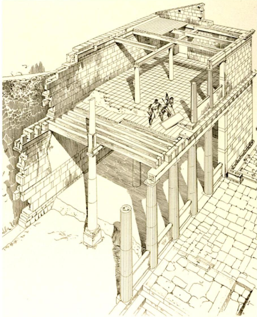
Şekil 45: Kuzey Stoa Alt ve Üst kat yapı elemanlarının kesitleri (Clarke, Bacon, Koldewey 1902: 45,1)
