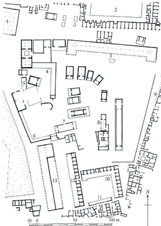
Şekil 37: Delos, Apollon Kutsal Alanı (J. J Coulton 1976, Fig.60)
