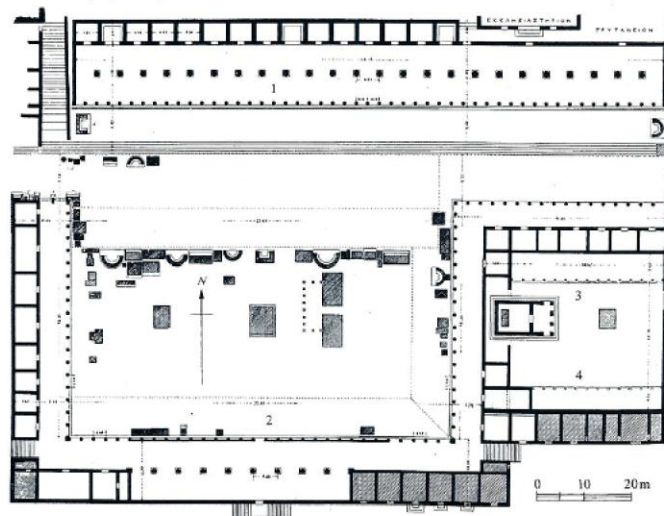
Şekil 29: Priene Agorası (J. J Coulton 1976, Fig.103)
