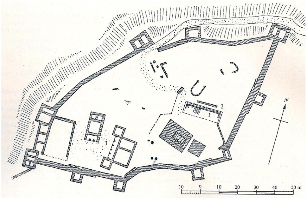
Şekil 4: Hermos, Larisa İ.Ö. 5.yy Akropolis Planı (J. J Coulton 1976, Fig.77) 1.Kuzey Stoa I 2.Kuzey Stoa II 3.Erken Dönem Sarayı
