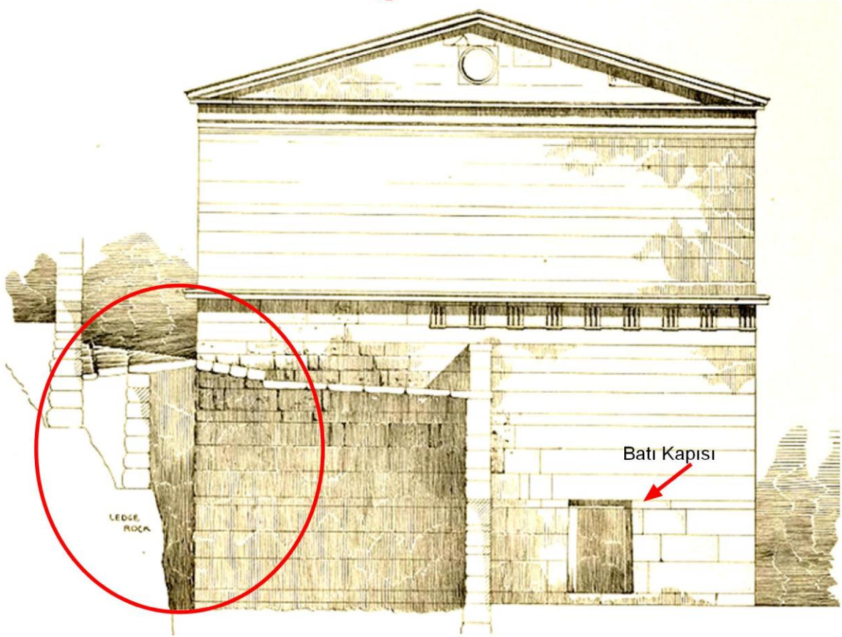
Şekil 42: Stoa batı kesiti. Batı Kapısı, Arka Duvarlar ve ara boşluk (Clarke, Bacon, Koldewey 1902: 41)
