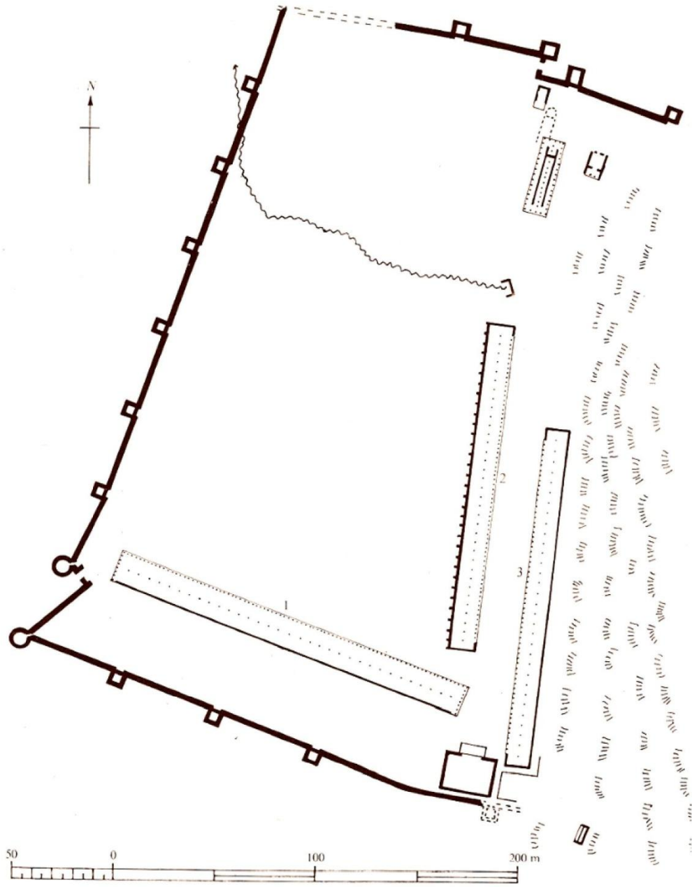
Şekil 35: Thermon Apollon Kutsal Alanı (J. J Coulton 1976, Fig.119) 1.Güney Stoa 2.Orta Stoa 3.Doğu Stoa
