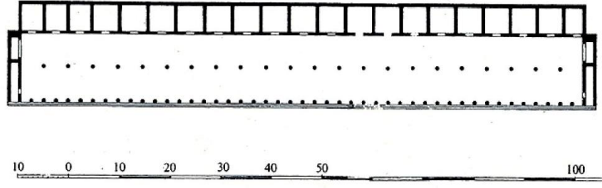
Şekil 34: Atina, Attalos Stoası (J. J Coulton 1976, Fig.24)
