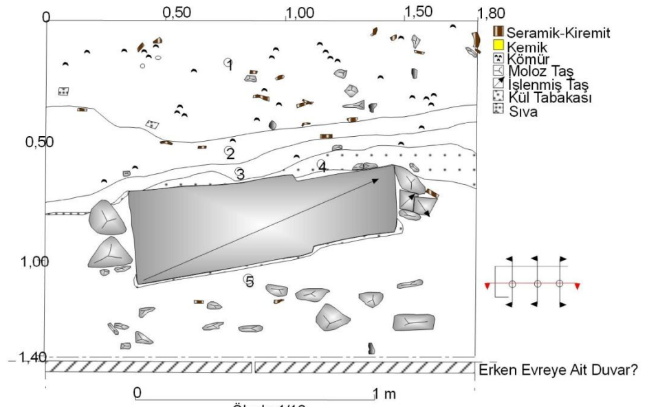
Şekil 61: Kuzey Stoa Alan 1 Profil 8 - Güney Profili
