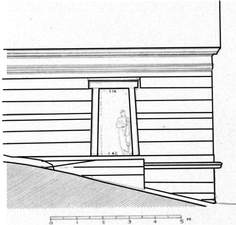
Şekil 46: Üst Kat batı Kapısı (Clarke, Bacon, Koldewey 1902: 49,2)
